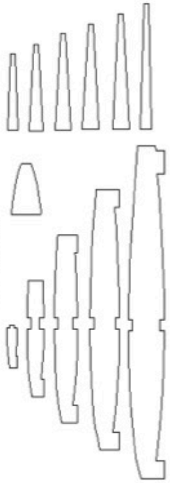
Fin / Rudder parts 3/32" Balsa
